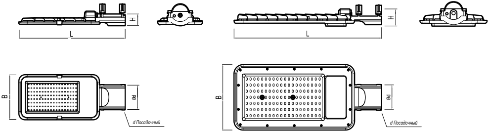
Рис 1. Светильник PSL 08 120°.
